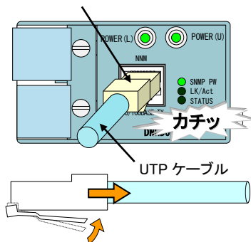
RJ-45 モジュラーコネクタ
