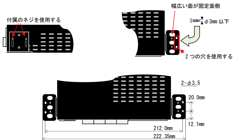
図 ねじによる固定方法
