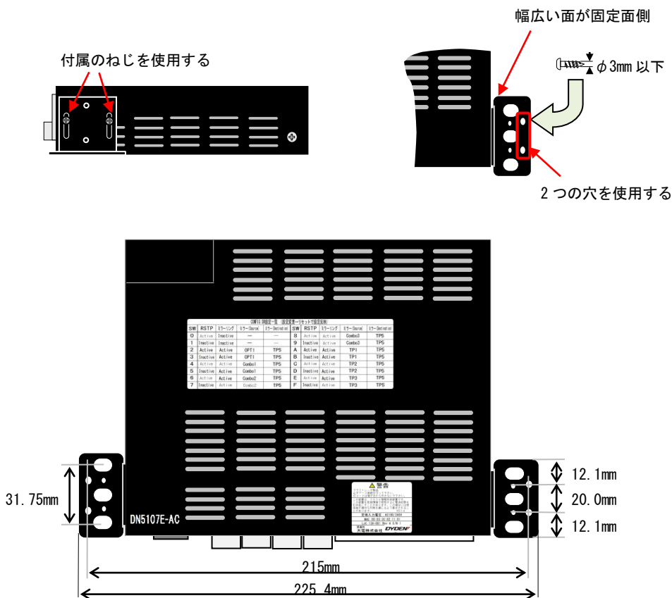
図 ねじによる固定方法
