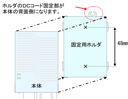
【ネジ固定時の下穴位置】
