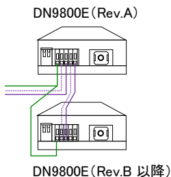
メタルケーブル接続 (NG)
