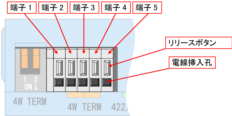
メタルポート端子配列
