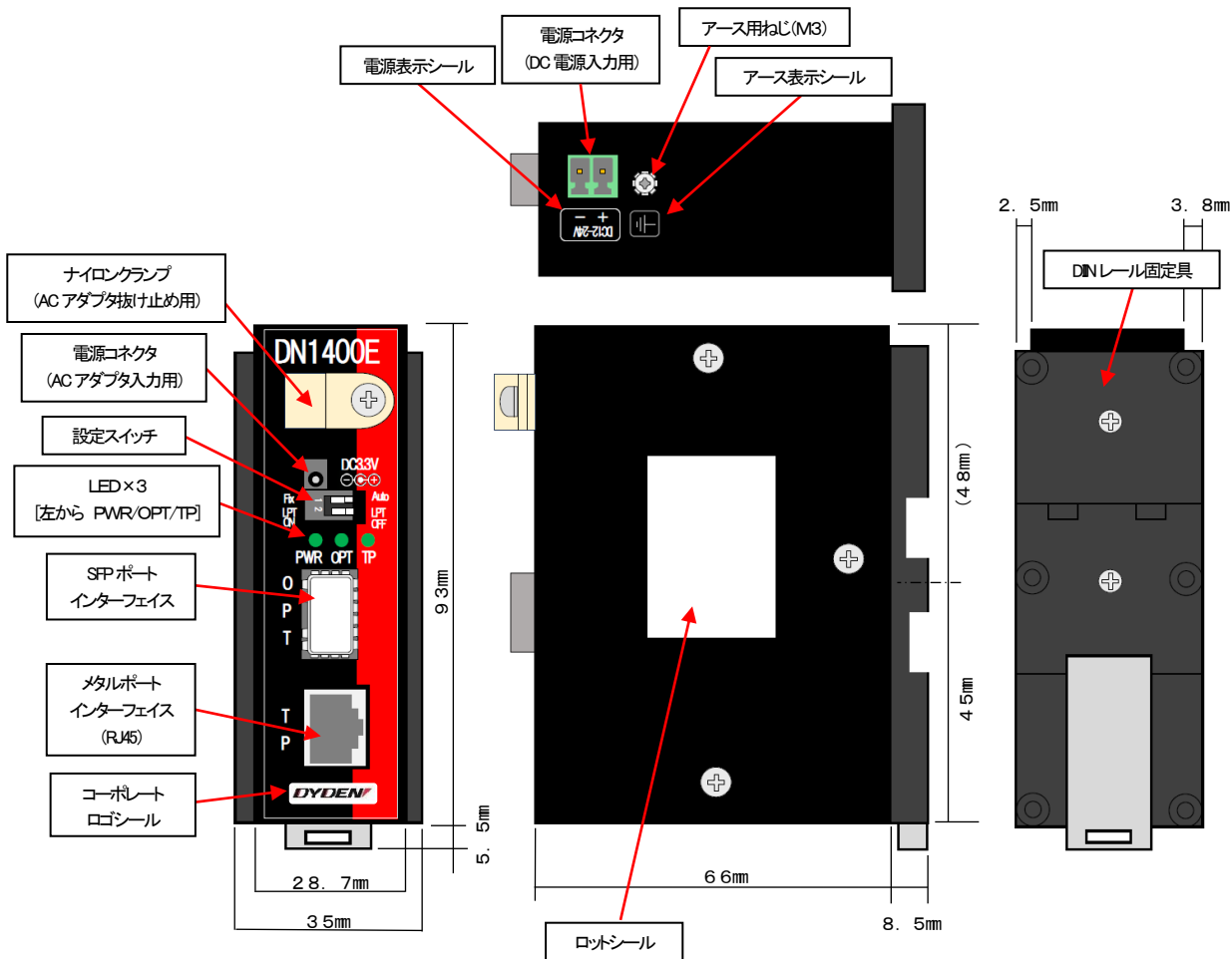
【外観図(筐体タイプ)】
