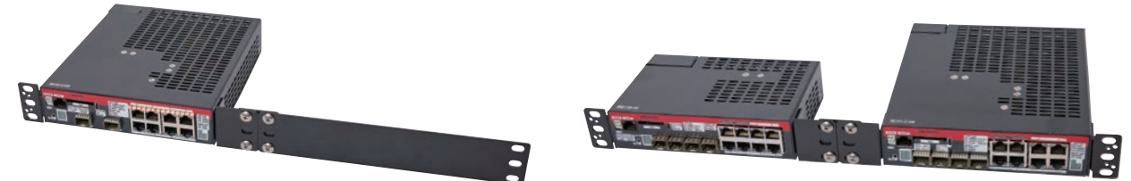
19インチラックに1台固定時(DNMB1E-42使用)
