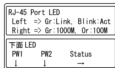
LED シール
