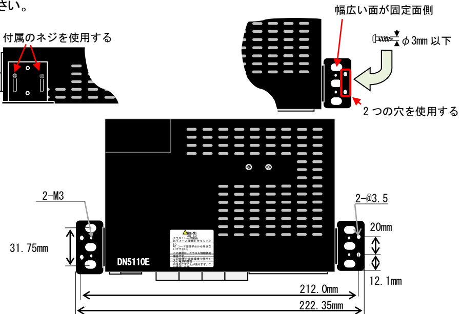
図 ネジによる固定方法
