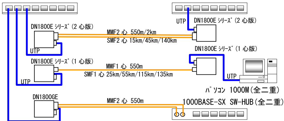
1000BASE-T SW-HUB(全二重)
