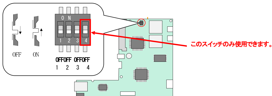
図 1.1 基板上的動作モード切り替えスイッチ
