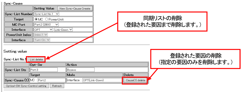
図 光バイパススイッチ同期リスト、要因の削除
