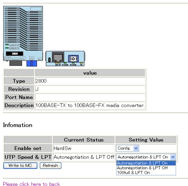
図 各ポート MC 設定画面
