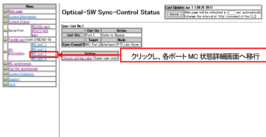
図 光バイパススイッチ同期機能表示画面 3
