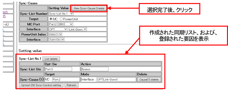
図 光バイパススイッチ同期要因登録 2
