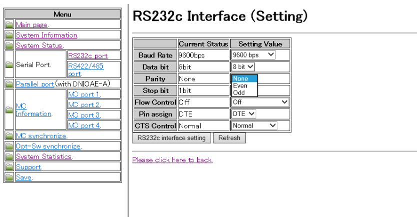
図 RS232c インターフェース設定画面
