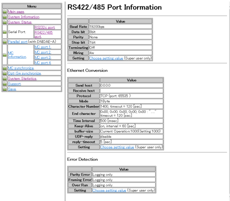
図 RS422/485 インターフェース、イーサ変換機能表示画面
