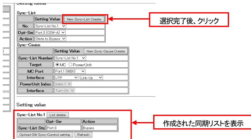
図 光バイパススイッチ同期リスト作成 2
